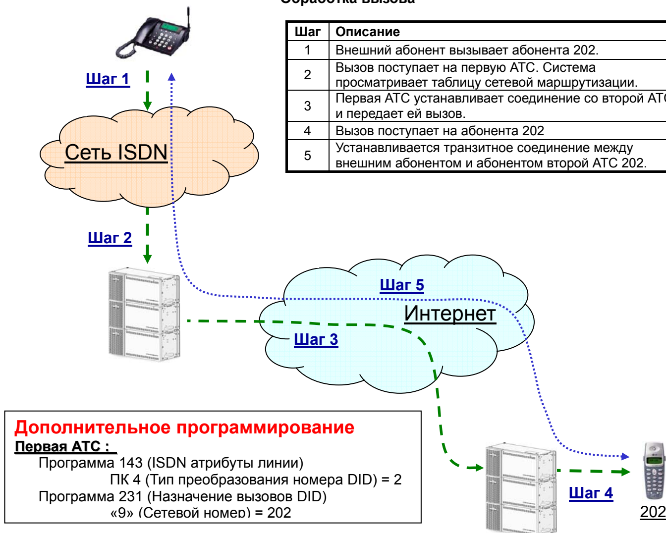
Рисунок 2.16.9 Обработка входящего внешнего вызова в сети АТС
